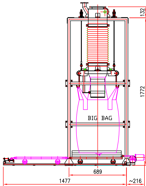
ELEVATION
