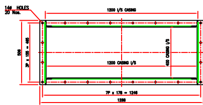
V.I.E.W : V2 V2 CASING FLANGE DETAIL
